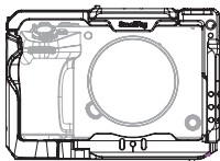
Front / 正视图
