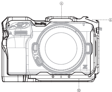
Front / 正视图
